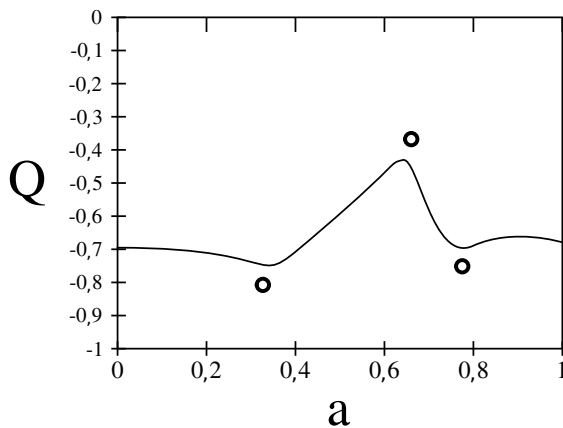
Figura 2.2: Ejemplo de wire-fitting . En esta imagen se muestra cómo los Q -valores de una acción unidimensional a son representados mediante una función continua definida mediante tres cables, mostrados como \circ .
